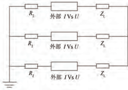
图 7 变压器二次侧电路结构
